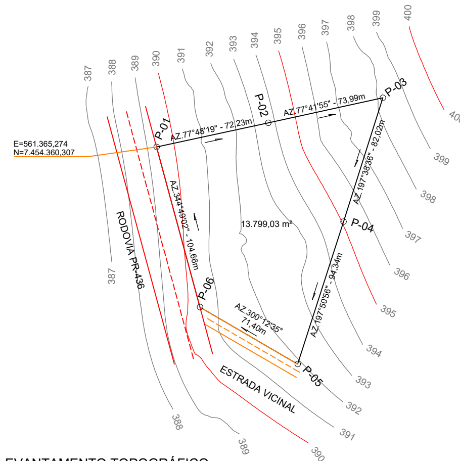
LEVANTAMENTO TOPOGRÁFICO
